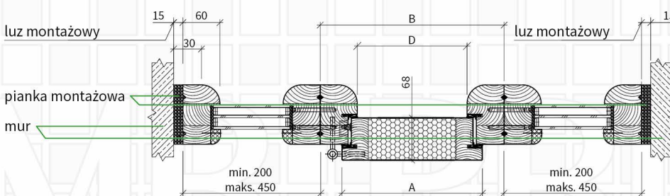
Przekrój poziomy drzwi z dwiema dostawkami
