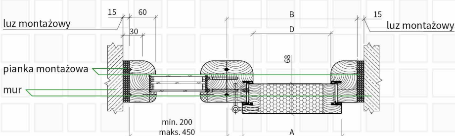
Przekrój poziomy drzwi z jedną dostawką
